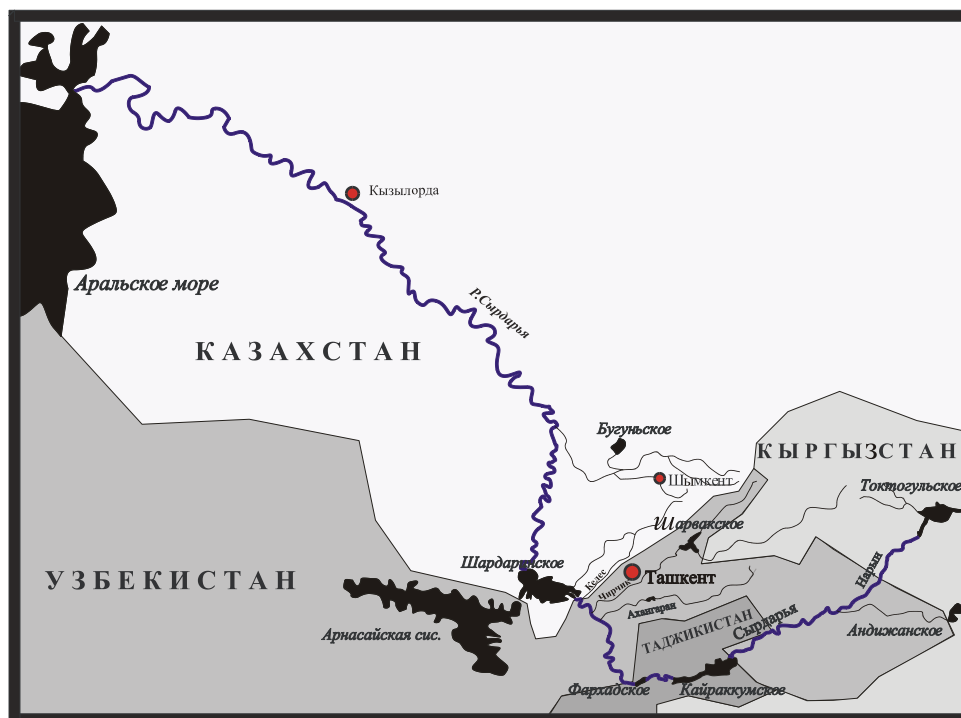
Рисунок 1. Схема бассейна реки Сырдарьи
