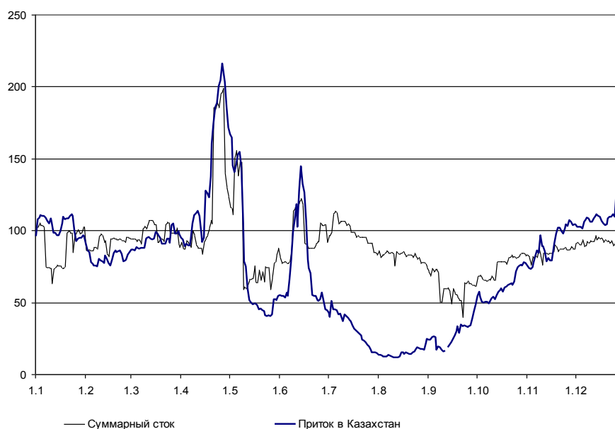
Рисунок 2. Сравнение притока воды в Казахстан с суммарным стоком Кайраккумского и Шарвакского водохранилищ (в млн.м³/сут. в течение года).
