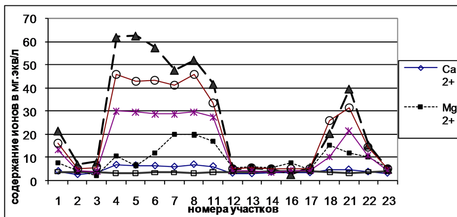
Рисунок 3. Качественный состав основных минеральных компонентов различных участков ДРУ
